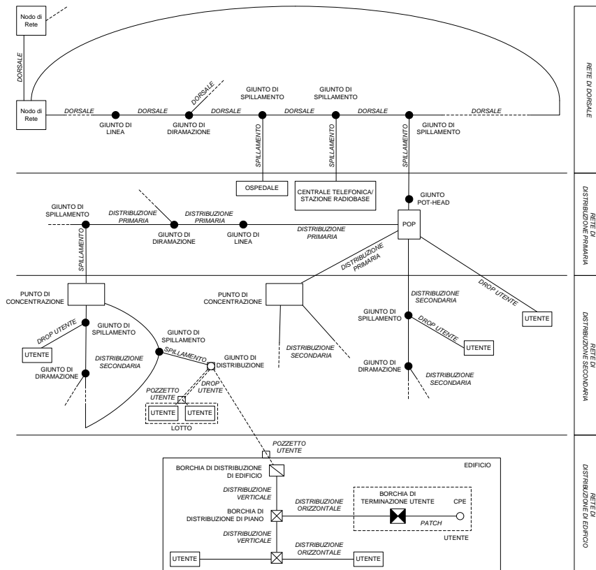
Figura 1 – Schema della rete
